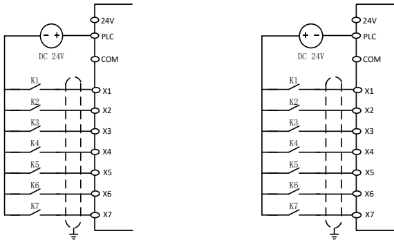
图 3-9 多功能输入端子接线图
