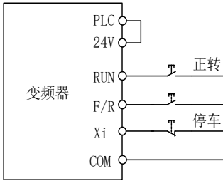
(a) F00.03=2 三线控制接线示意图
