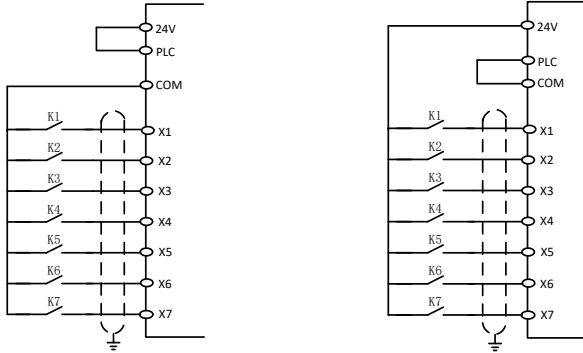
C、NPN 模式使用外部电源
