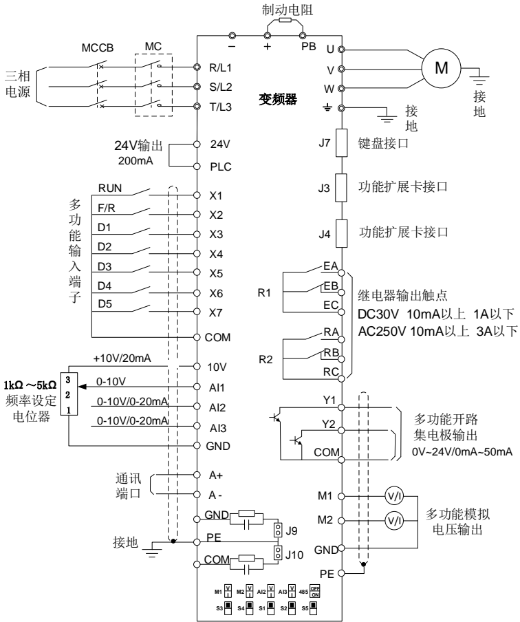
图 3-13 控制回路标准接线图
