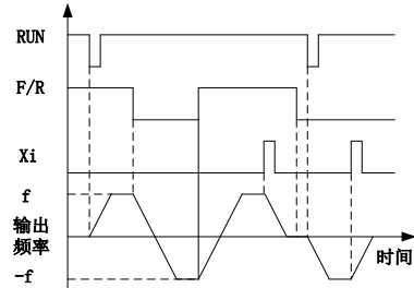
(d) F04.19=0, F00.03=3 正/反转运行逻辑
