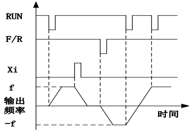
(b) F04.19=0, F00.03=2 正/反转运行逻辑
