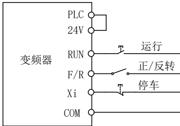
(c) F00.03=3 三线控制接线示意图
